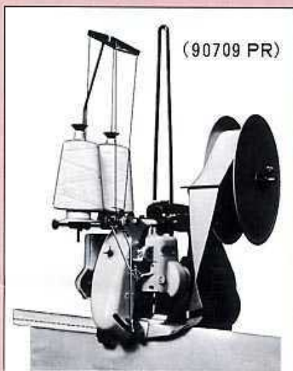
テーブルフォルダー及びカッターセット
